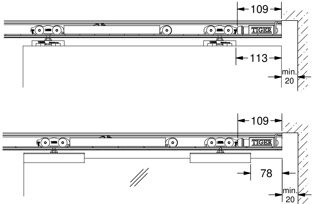
T-Master 150NOVA
